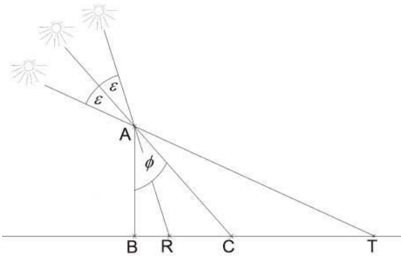
Abb. 295 Gnomonlänge AB und Schattenlängen, Winkel der Ortsbreite und der Eklipsenchiefe.
