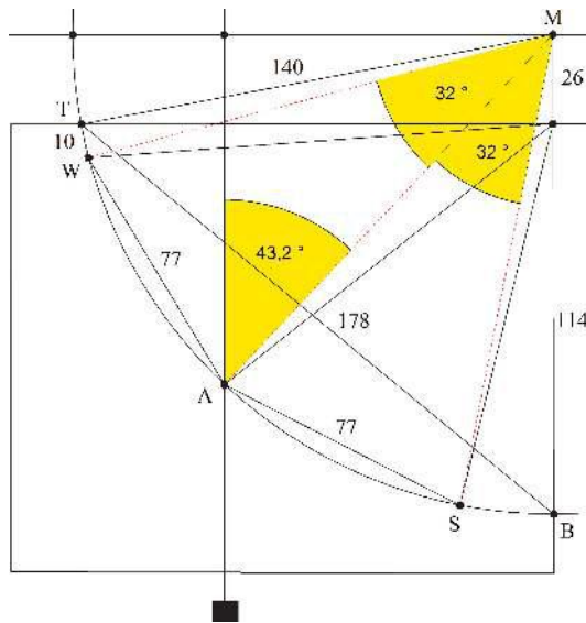
Abb. 348 i 57: Meridianebene ( M = G ).
