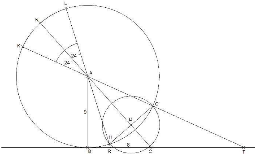
Abb. 298 Analemma des Vitruv.
