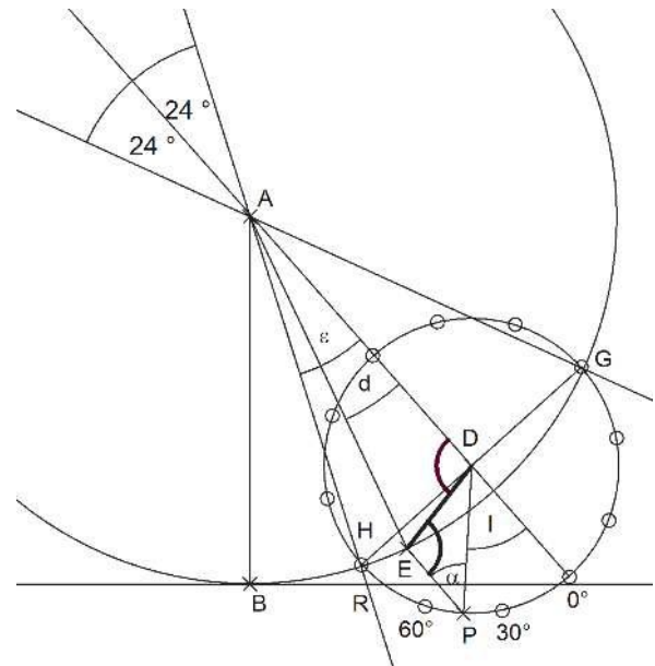
Abb. 300 Eklptikale Länge und Deklination am Manaeus.
