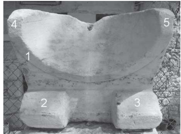
Abb. 131 Eine Hohlsonnenuhr und ihre Teile, gezeigt an ii 45 aus Samos (Form S 1 L).
