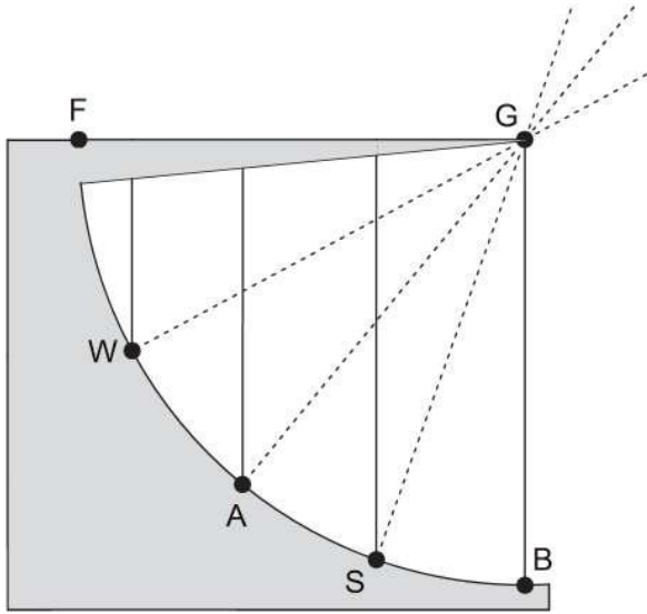
Abb. 306 Meridianebene einer Hohlkugelsonnenuhr mit Pseudodatumlinien. Die lang gestrichelten Datumsebenen liegen vertikal zur Horizontebene; Sonnenstrahlen sind durch kurze Striche angedeutet.
