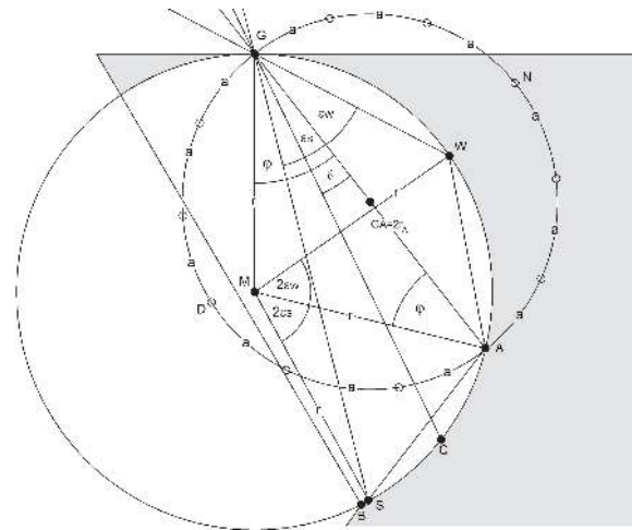
Abb. 310 ii 1: Meridianebene von Schattenfläche I mit Äquinoktialkreis.
